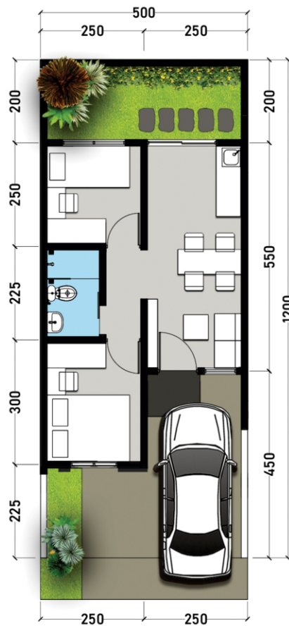
Denah Rumah
