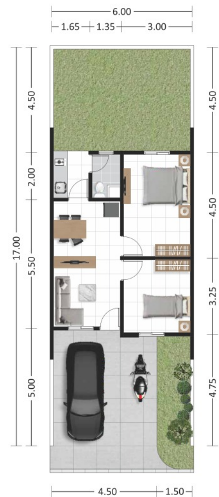
DENAH T.53
