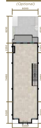
LANTAI 3
