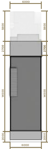
DAK ATAP
