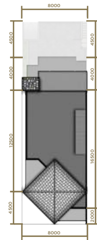
DAK ATAP
