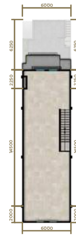
LANTAI 3
