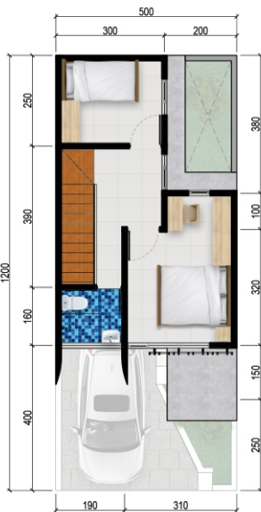
LANTAI 2
