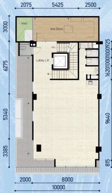
Lantai 2
