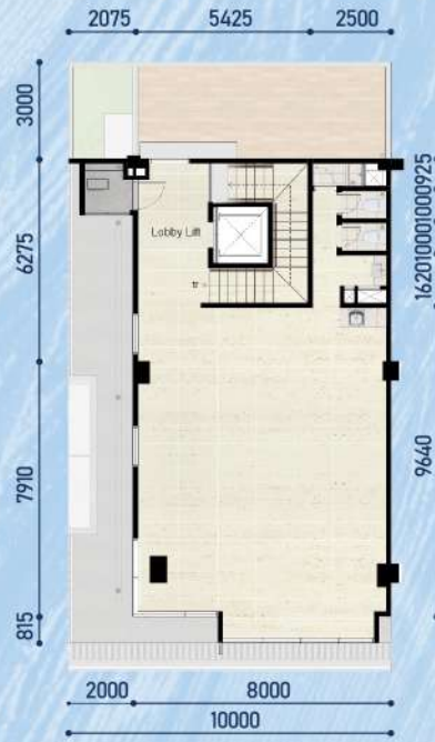
Lantai 3
