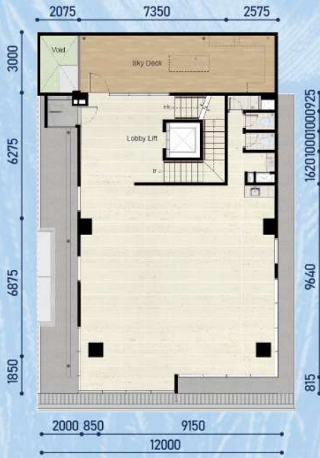
Lantai 2
