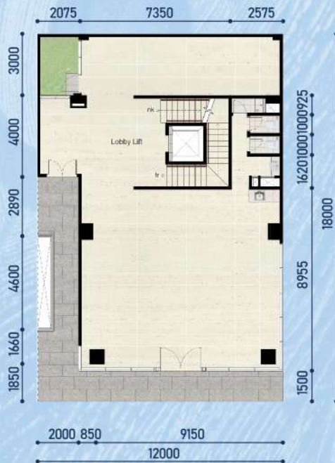
Lantai Dasar
