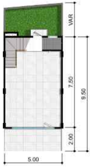
DENAH LT.1
