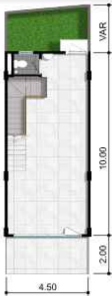
DENAH LT.1
