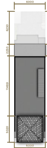
DAK ATAP
