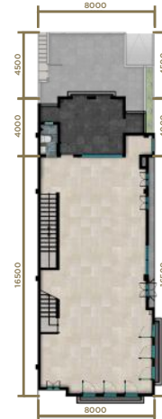
LANTAI 2
