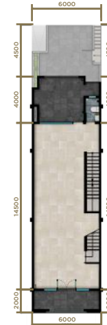
LANTAI 2
