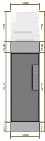
DAK ATAP
