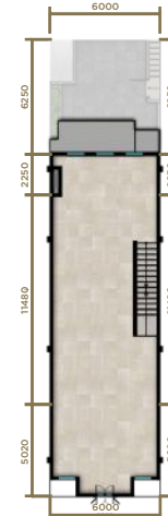
LANTAI 3
