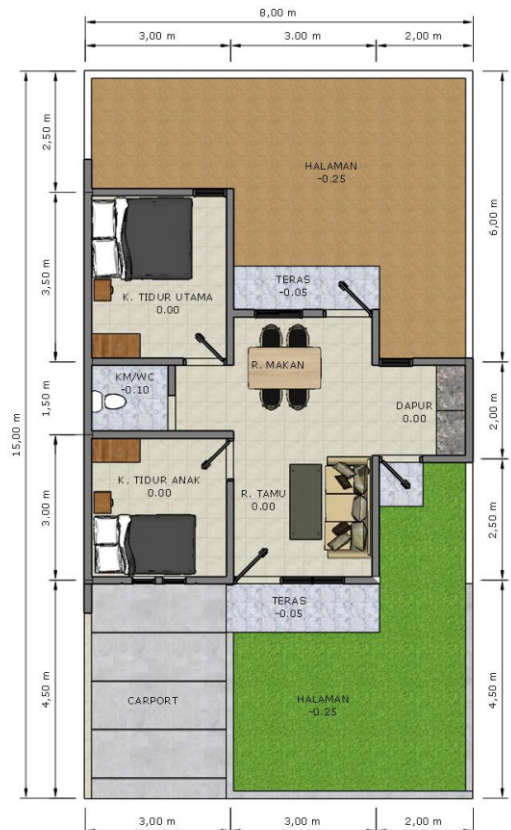
DENAH TIPE 45/120 *Tanpa Pagar Keliling
