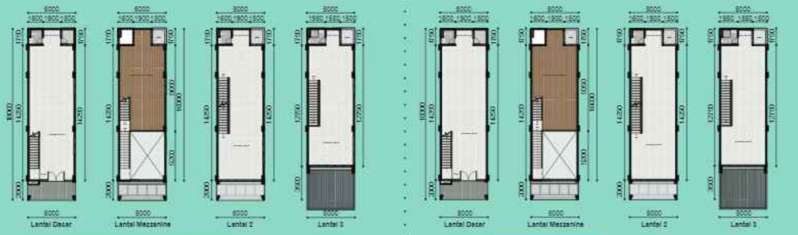
5 X 17 Meter LT: 85 LB: 247 | 5 X 18 Meter LT: 90 LB: 278
