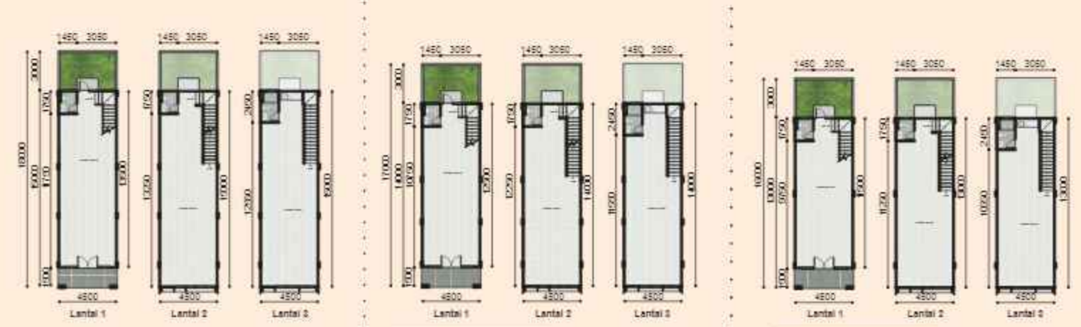
4,5 X 18 Meter LT: 81 LB: 203 | 4,5 X 17 Meter LT: 76,5 LB: 190 | 4,5 X 16 Meter LT: 72 LB: 176
