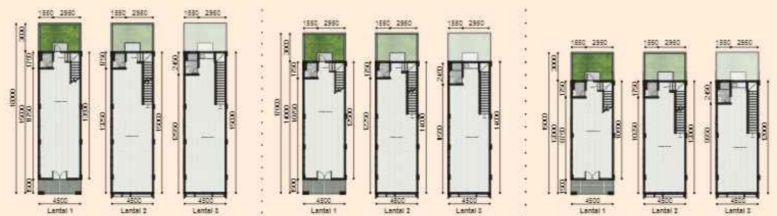
4,5 X 18 Meter (CORNER TYPE) LT: 81 LB: 203 | 4,5 X 17 Meter (CORNER TYPE) LT: 76,5 LB: 190 | 4,5 X 15 Meter (CORNER TYPE) LT: 67,5 LB: 163
