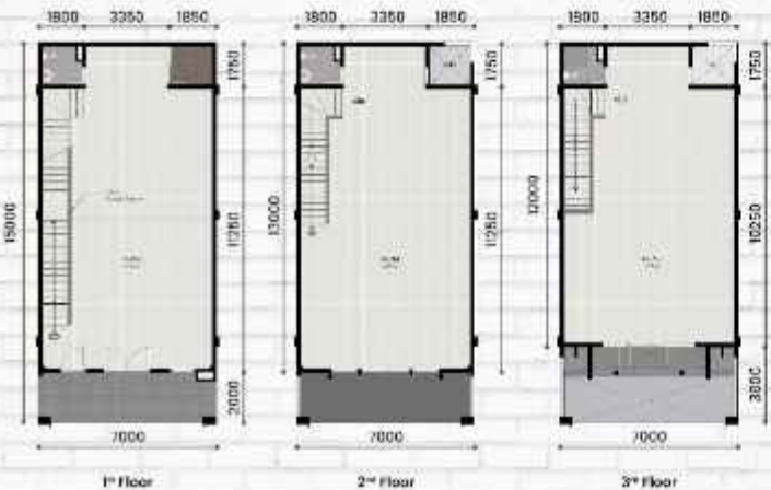
Standard Type 7 x 15 LT : 105 m 2 | LB : 268 m 2
