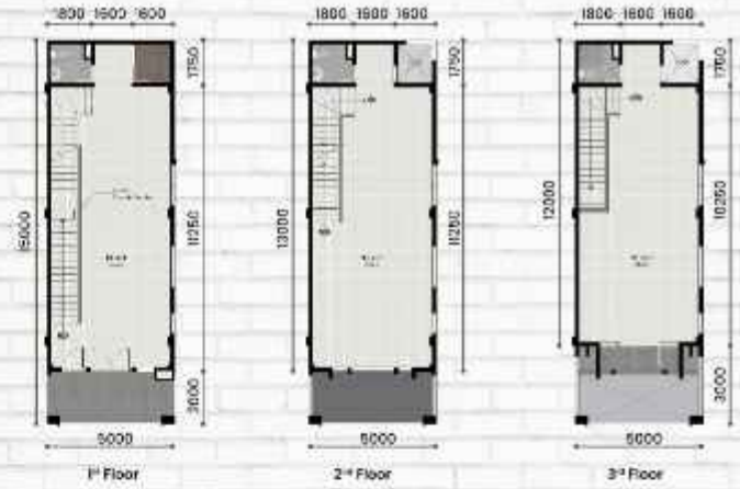
Hoek Type 5 x 15 LT : 75 m 2 | LB : 190 m 2
