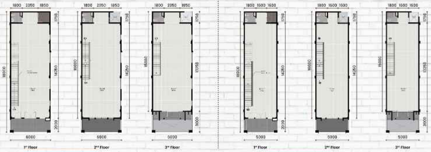
Standard Type 6 x 18 LT : 108 m 2 | LB : 282 m 2
