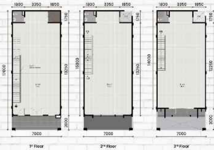
Standard Type 7 x 17 LT : 119 m 2 | LB : 310 m 2
