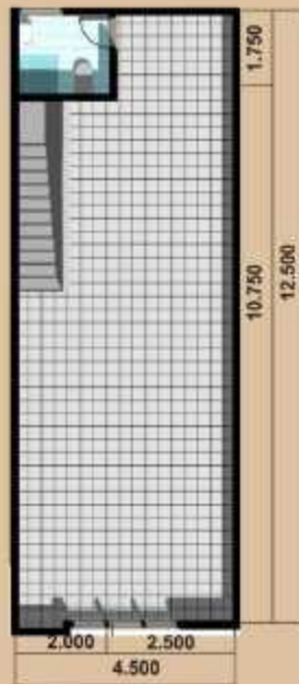
DENAH LANTAI ATAS
