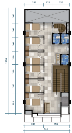
LANTAI 2 (Alternatif Pengembangan Rukos) Dinding penyekat, hanya berupa ilustrasi. Informasi lebih lanjut hubungi bagian Konsultasi Desain
