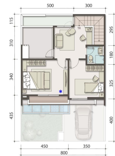
LANTAI 2
