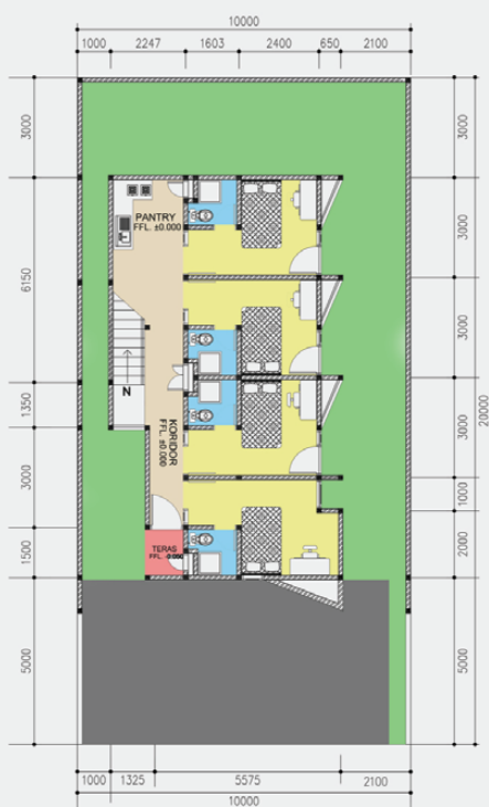
LANTAI DASAR
