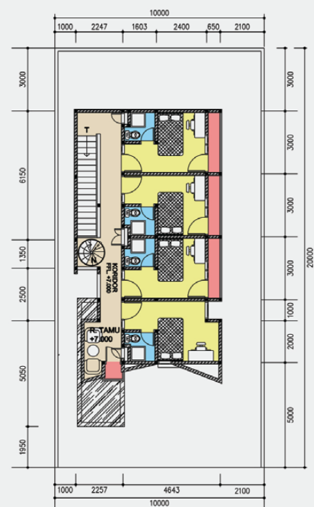
LANTAI DUA
