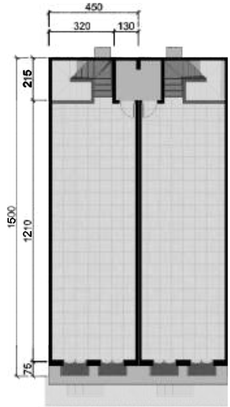
Lantai Atas
