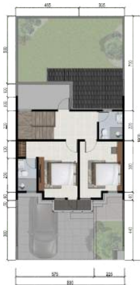
Lantai Atas
